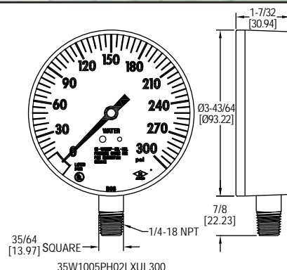
35W1005PH02LXUL300
